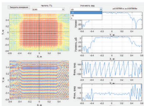
АФР, измеренное в ближней зоне
