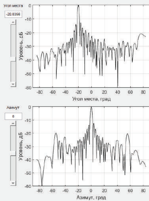
АФР, восстановленное на плоскости АФР с отказавшим элементом
