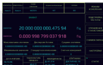
Главное окно встроенного программного обеспечения
