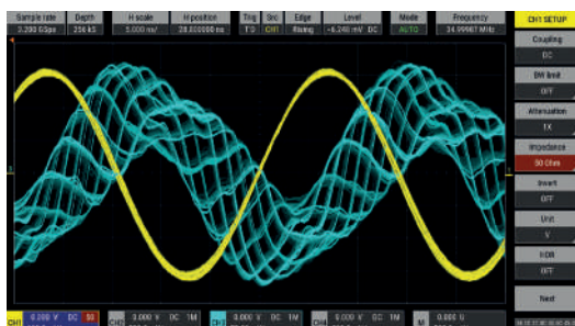
Пример отображения сигналов осциллографом в двухканальном режиме
