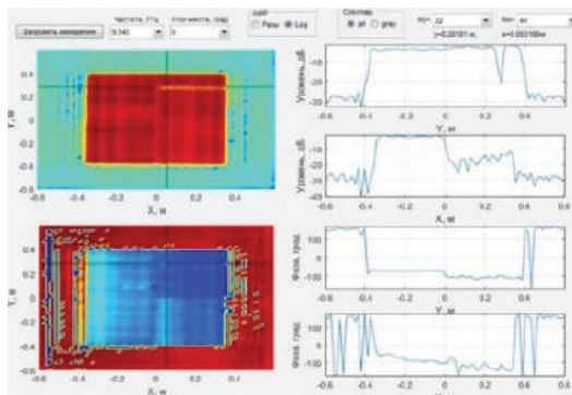
АФР, восстановленное на плоскости АФР с отказавшим элементом
