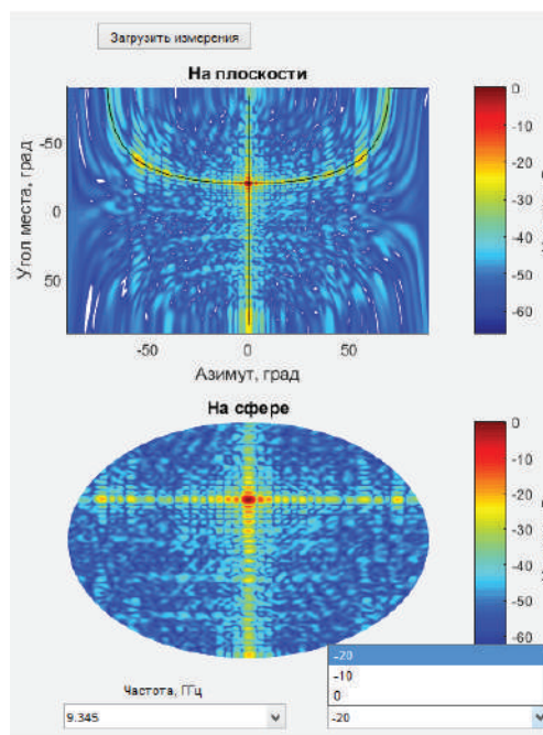
АФР, измеренное в ближней зоне
